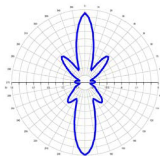
E-Plane
